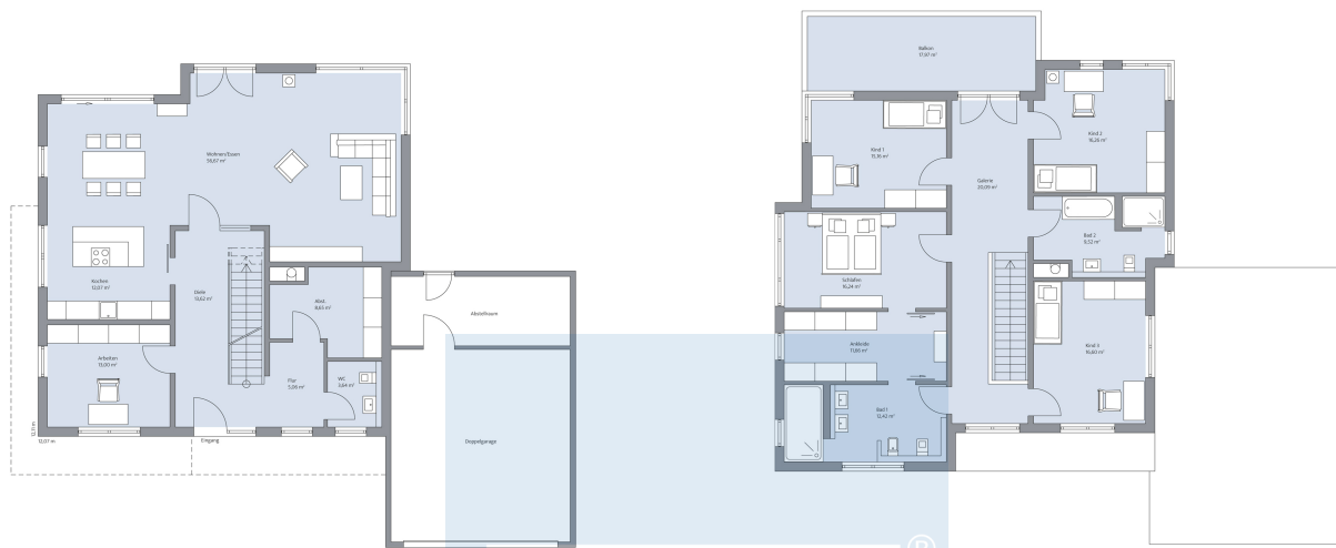
Haus Campmann Grundriss EG
