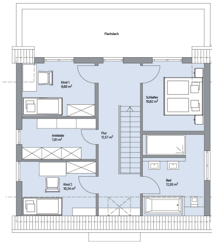
Haus Tesche Grundriss
