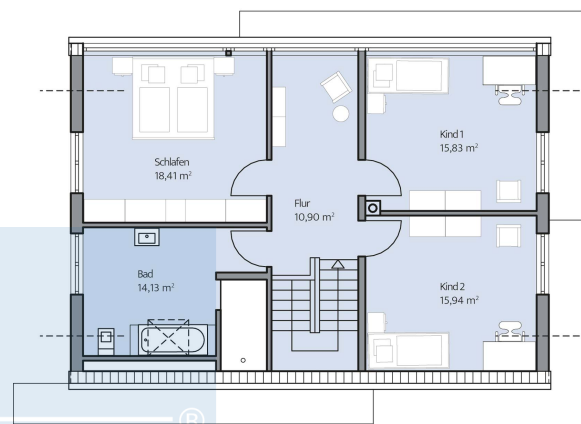
Haus Vettel Grundriss
