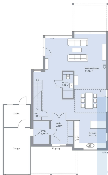
Haus Hildebrand Grundriss
