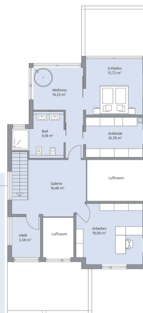
Haus Hildebrand Grundriss
